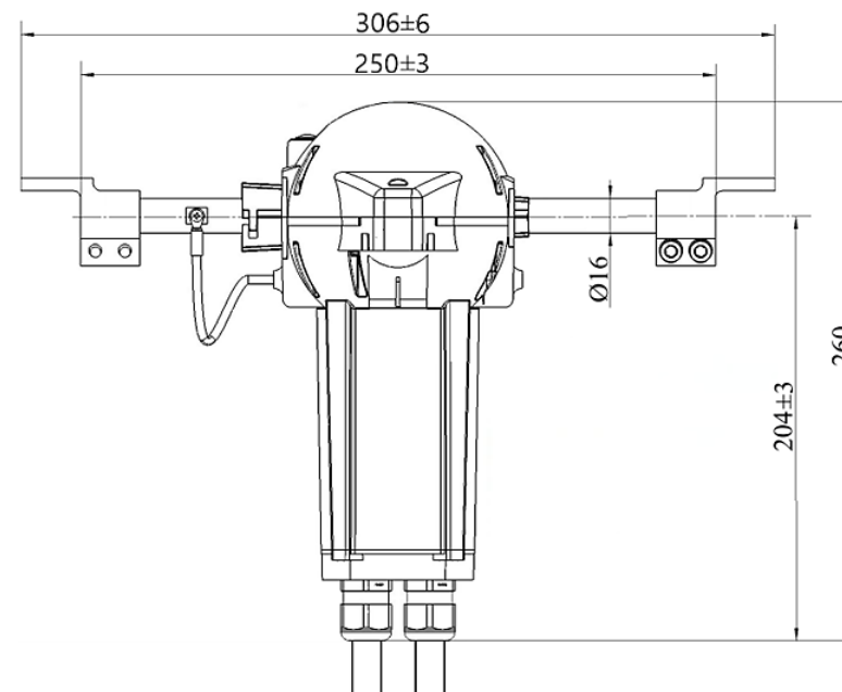
БЛОК СОЕДИНИТЕЛЬНЫЙ
